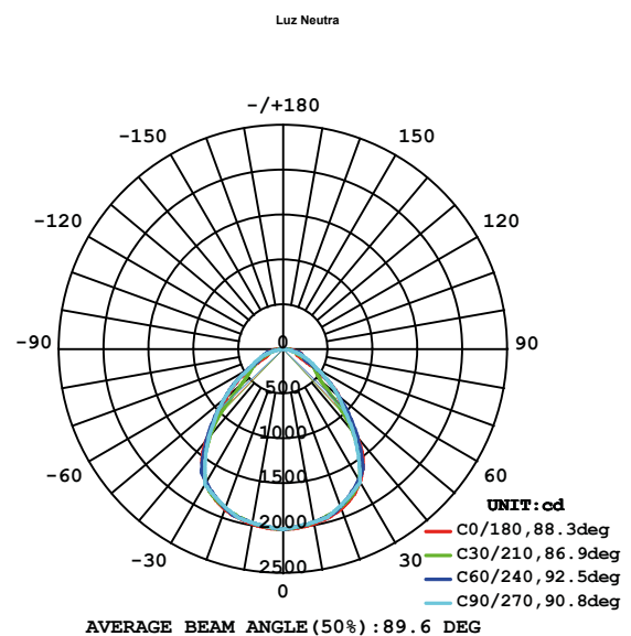
Curva de Distribución Lumínica
