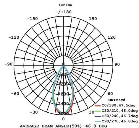
Curva de Distribución Lumínica
