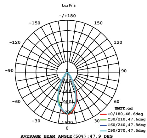
Curva de Distribución Lumínica
