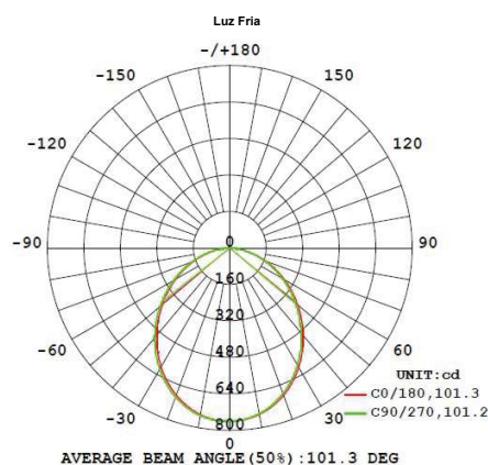
Curva de Distribución Luminosa
