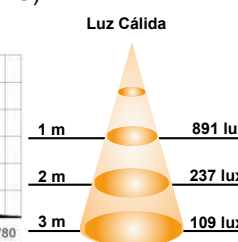
Curva de Distribución Luminosa
