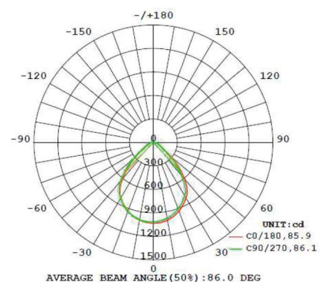
Curva de Distribución Lumínica
